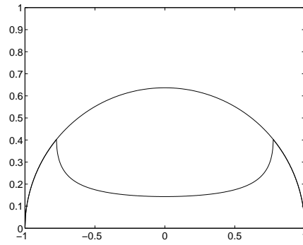
(d) Constraint \sigma and theoretical solution t\mu_t of 4.1.2
